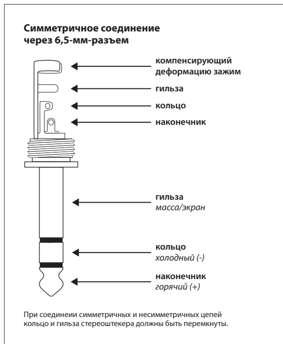
Рис. 4.3: 6,3 мм- стереоштекер
