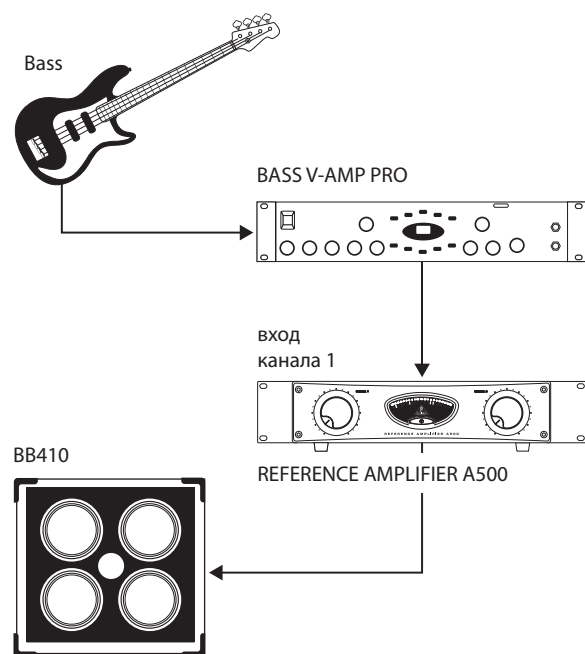
Рис. 3.2: Мостовой режим
