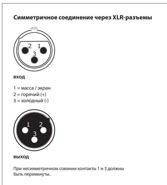
Рис. 4.1: Разъемы XLR
