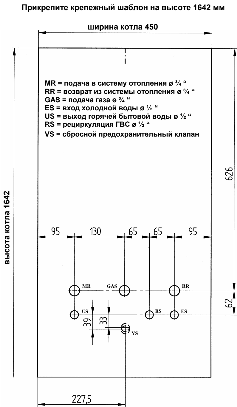
Рис.2 Крепежный шаблон COMBI
