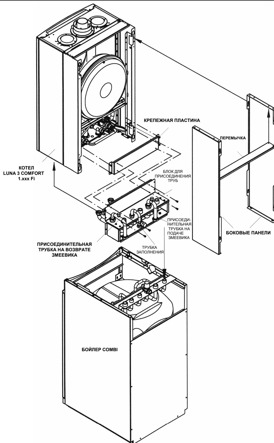
Рис. 1А Последовательность операций по присоединению бойлера
