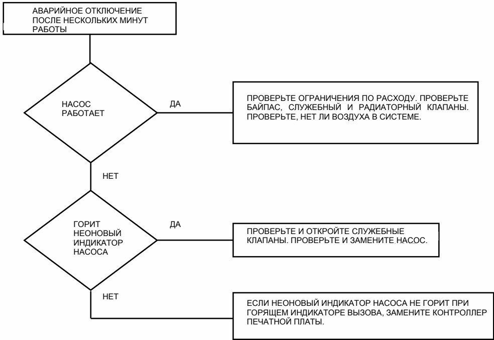
РИС. 19 АВАРИЙНЫЙ СИГНАЛ 3
