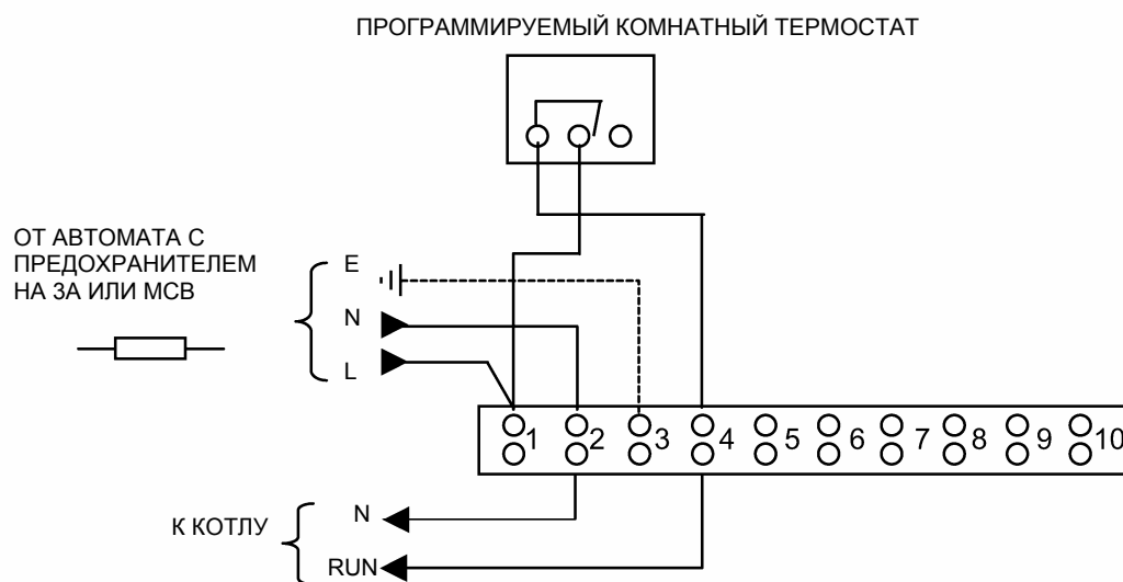
РИС. 10 ТИПИЧНАЯ ЭЛЕКТРИЧЕСКАЯ СХЕМА ПРИ ИСПОЛЬЗОВАНИИ КОТЛА ТОЛЬКО ДЛЯ ОТОПЛЕНИЯ
