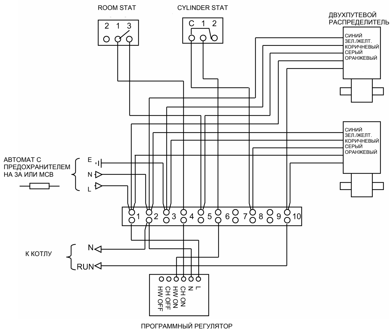
РИС. 8 ТИПИЧНАЯ ЭЛЕКТРИЧЕСКАЯ СХЕМА S PLAN
