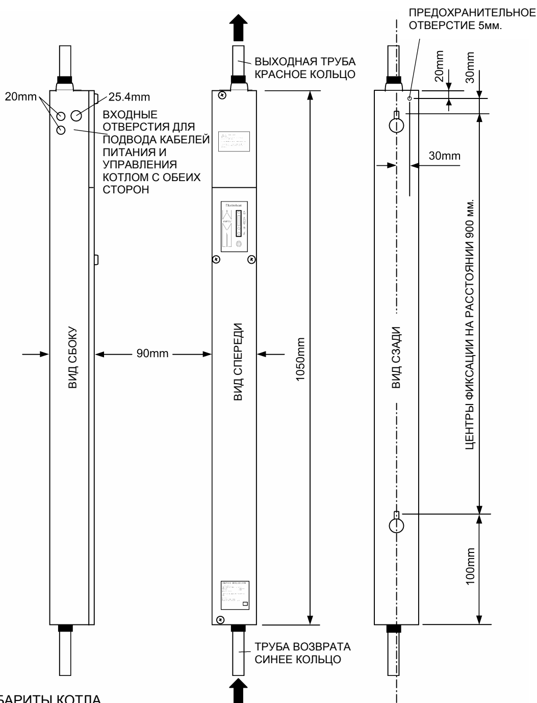
РИС. 2 ГАБАРИТЫ КОТЛА
