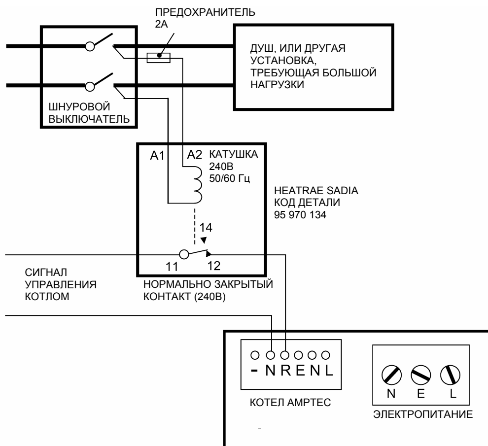
РИС. 24 РЕЛЕЙНАЯ РЕГУЛИРОВКА ДУША
