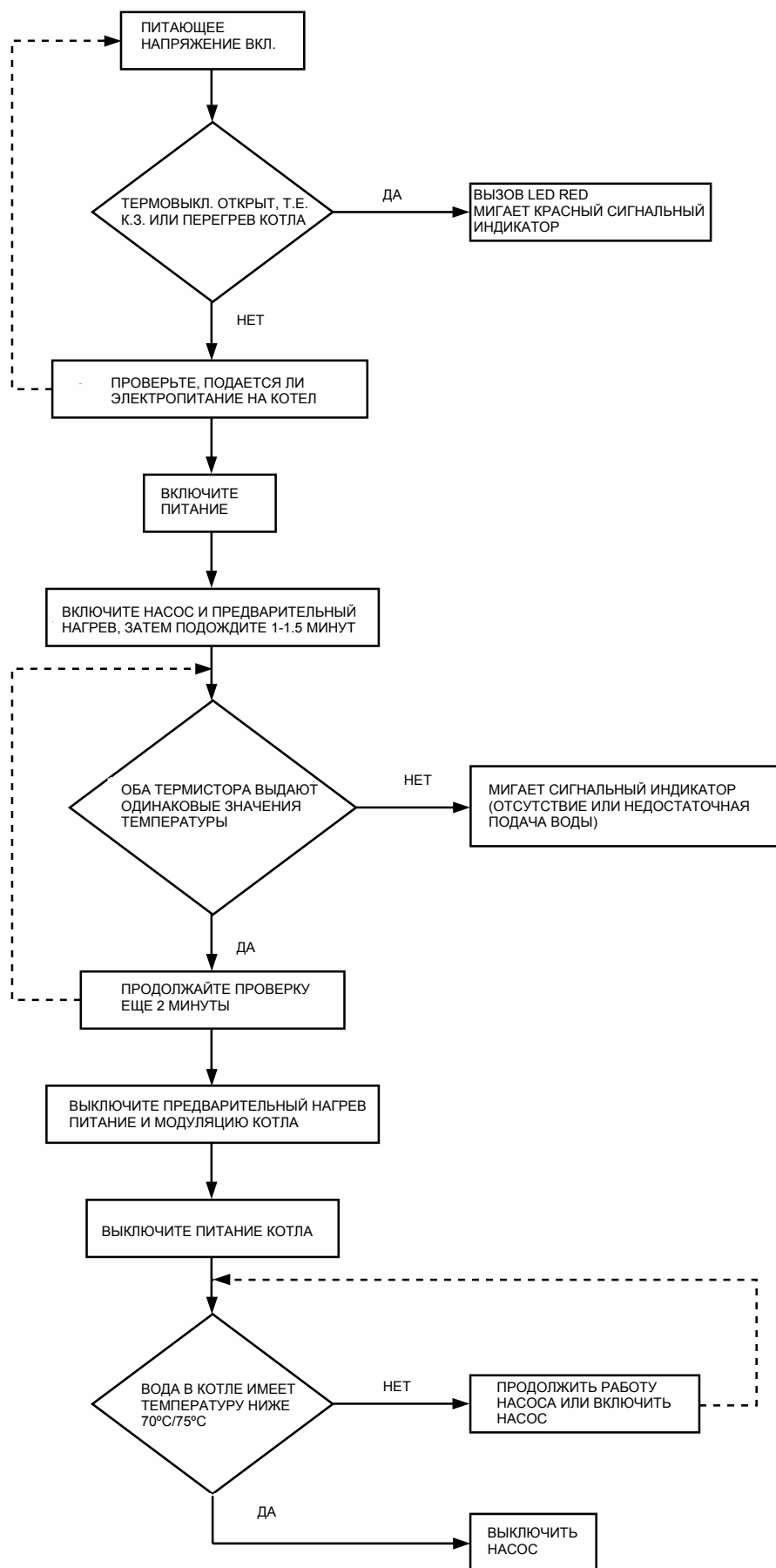
РИС. 12 РАБОТА КОТЛА СЕРИИ С ВЫПУСКА 5
