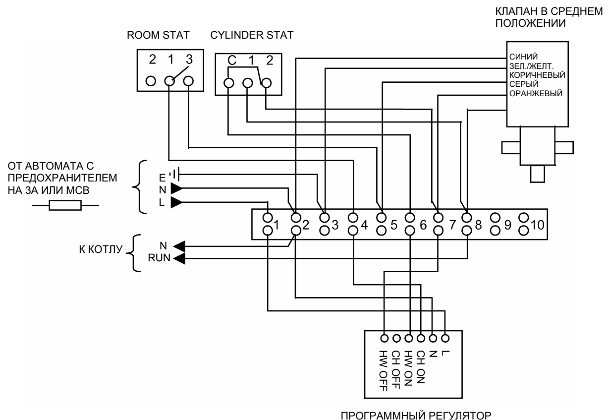
РИС. 9 ТИПИЧНАЯ ЭЛЕКТРИЧЕСКАЯ СХЕМА Y PLAN
