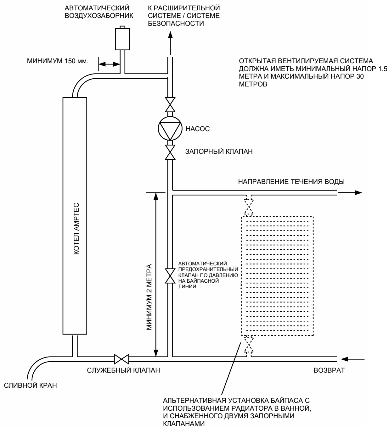
РИС. 3 ГЛАВНАЯ СХЕМА ВОДОСНАБЖЕНИЯ
