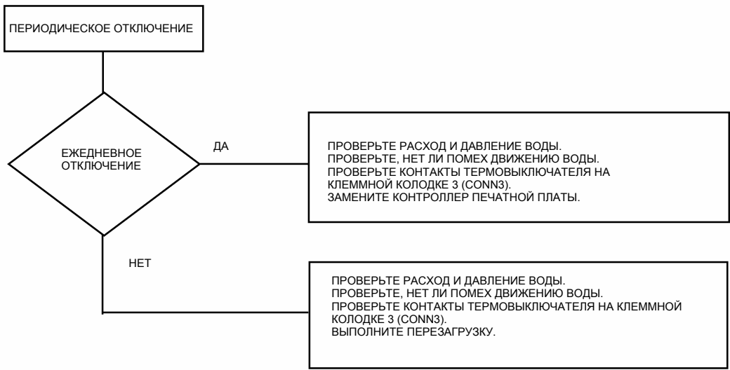
РИС. 20 АВАРИЙНЫЙ СИГНАЛ 4
