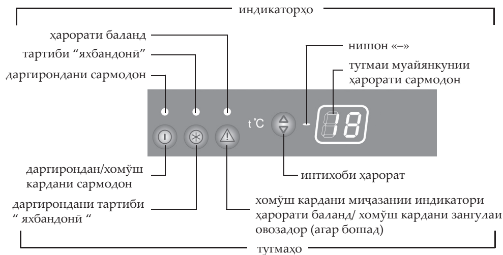
Рисми 3 – Ғалтаки идоракунии
