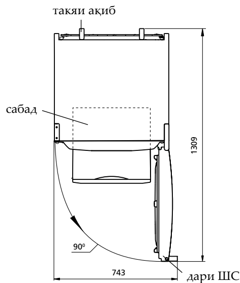
Расми 2 – Яҳдон (намои болоӣ)
