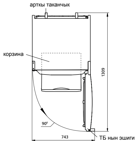
2-сүрөт – Муздаткыч (үстүнөн караганда)
