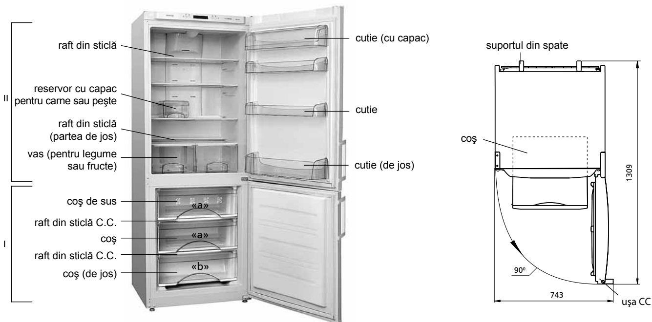
Figura 2 – Frigiderul (privire de sus)
