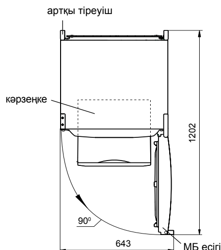
2-сурет – Тоңазытқыш (үстінен қарау)
