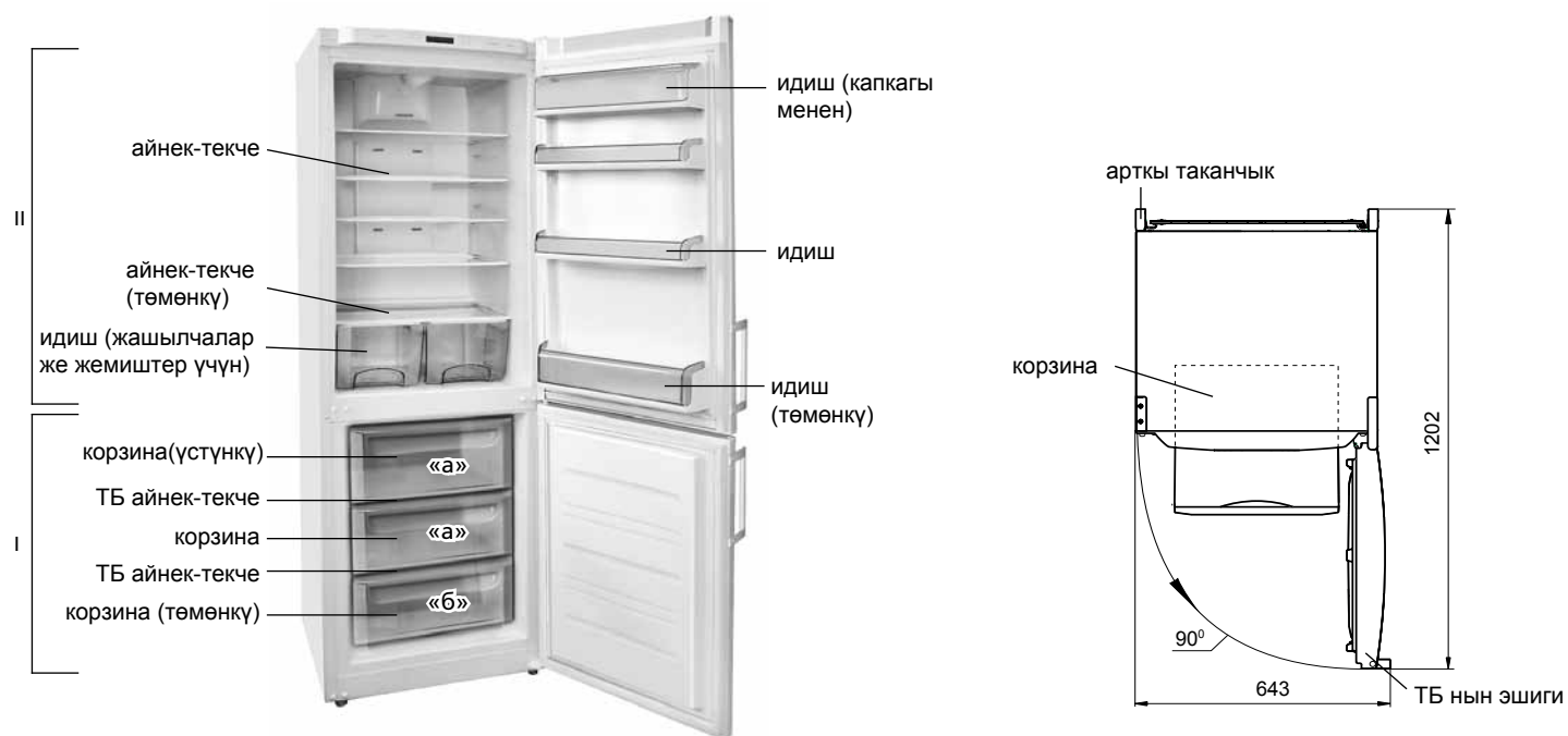
2-сүрөт – Муздаткыч (үстүнөн караганда)
