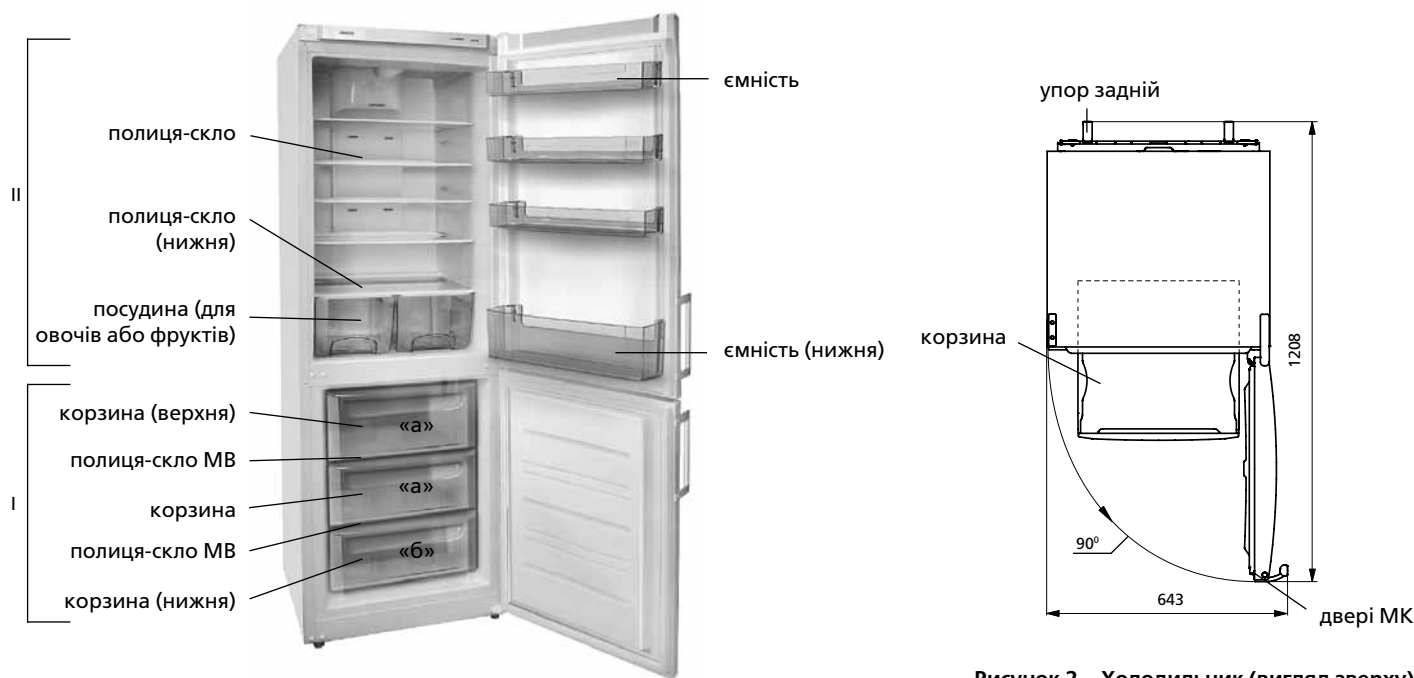
Рисунок 2 – Холодильник (вигляд зверху)
