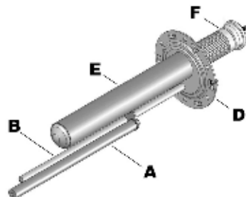
Рис. 2. Стоечатый нагревательный элемент + магниевый анод
